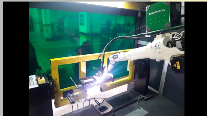
Tel beslemeli robotik TIG kaynak sistemi
